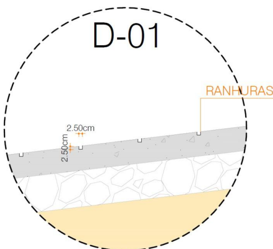
Figura 9 - – Detalhe das ranhuras da rampa náutica de concreto. Fonte: São Paulo (2021) apud Brasil (2024). Elaboração: LabTrans/UFSC (2022).
