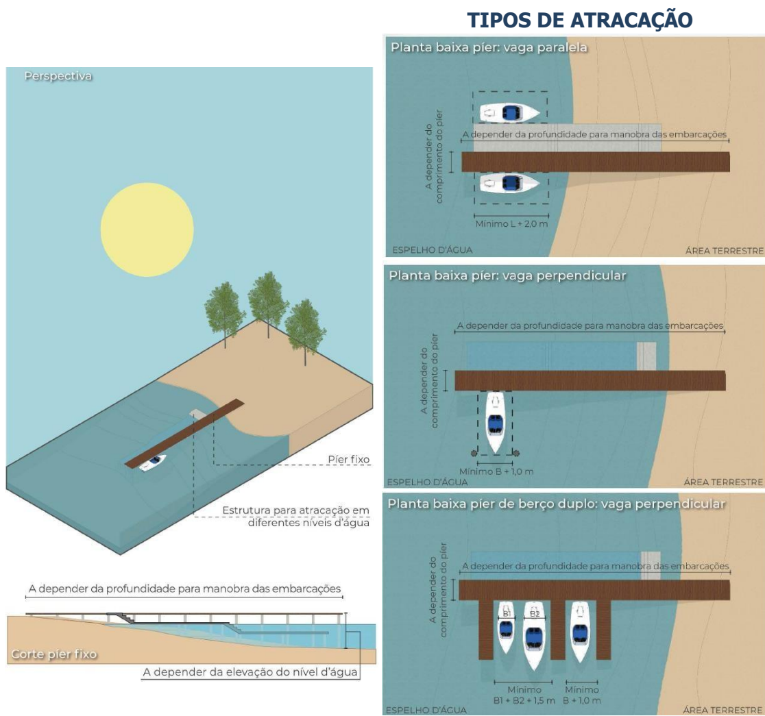
Figura 12- Representação das Recomendações técnicas para píeres fixos. Fonte: Brasil (2024). Elaboração: LabTrans UFSC (2023).
