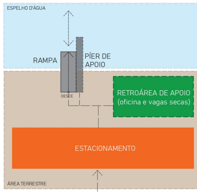
Figura 5 - Programa de necessidades da rampa náutica. Fonte: Brasil (2024). Elaboração: LabTrans/UFSC (2022).
