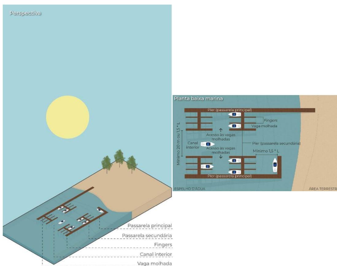
Figura 15 - Representação das Recomendações técnicas para marinas. Fonte: Brasil (2024). Elaboração: LabTrans UFSC (2023).
