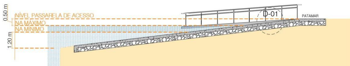
CORTE AA - RAMPA NÁUTICA
