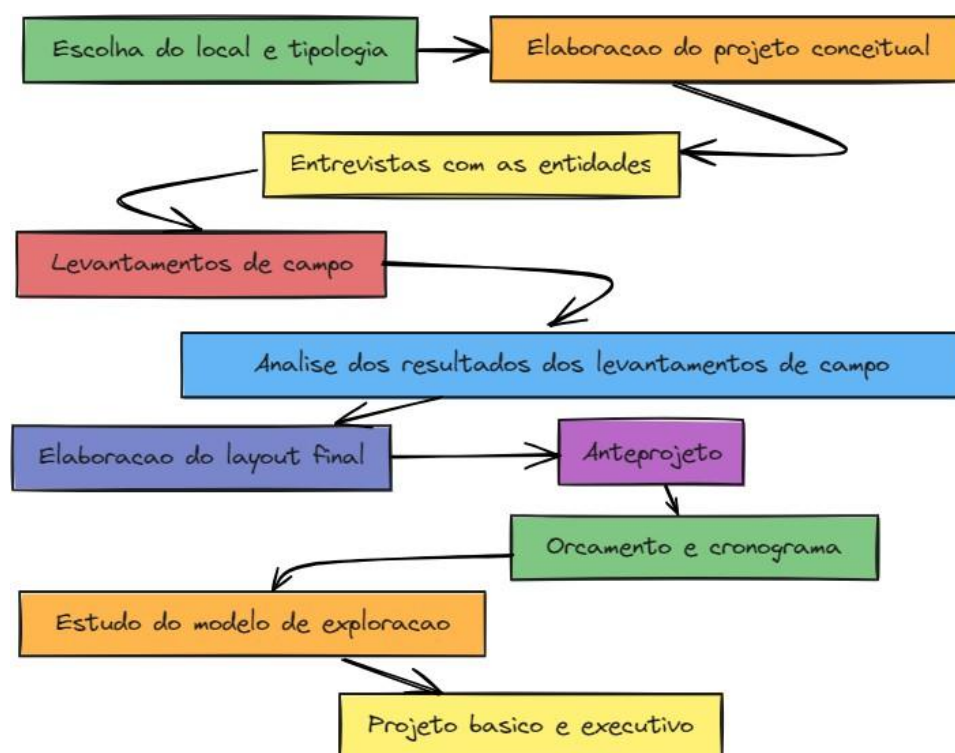
Figura 4 – Fluxograma das etapas de trabalho para elaboração dos anteprojetos e dos modelos de exploração. Fonte: Brasil (2024). Elaboração Própria.
