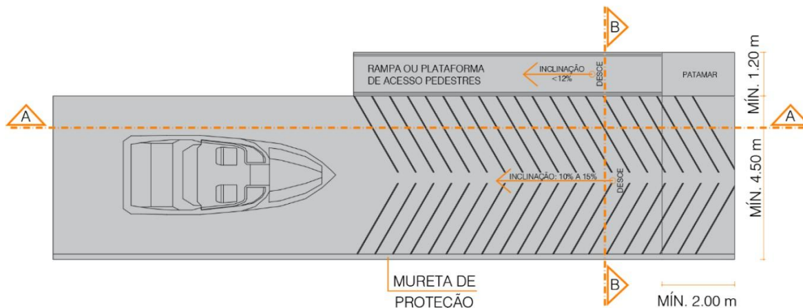
Figura 6 - Planta baixa do projeto conceitual de uma rampa náutica.
