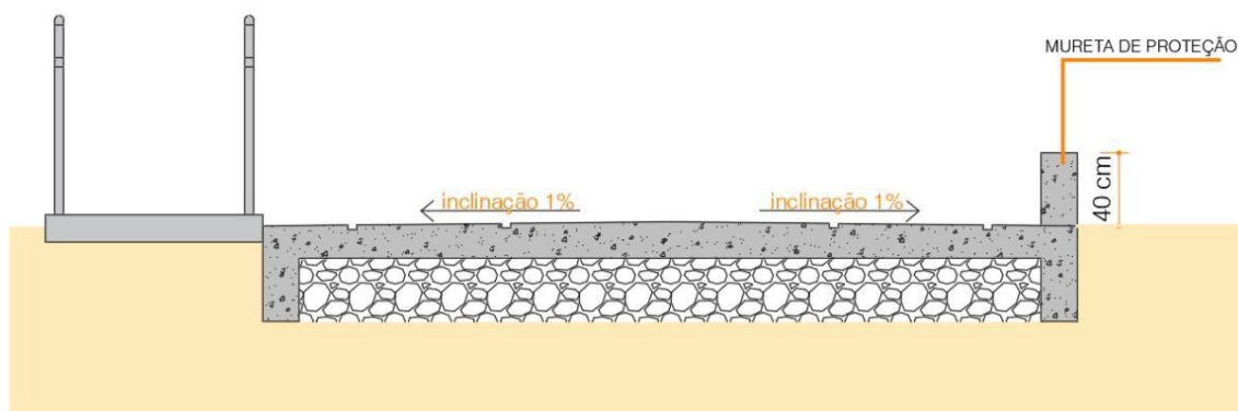
Figura 7 - Seção longitudinal do projeto conceitual de uma rampa náutica. Fonte: São Paulo (2021) apud Brasil (2024). Elaboração: LabTrans/UFSC (2022).
