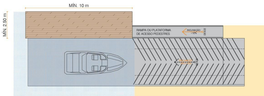
Figura 10 -- Conjunto de rampa náutica com píer de apoio. Fonte: São Paulo (2021) apud Brasil (2024). Elaboração: LabTrans/UFSC (2022).
